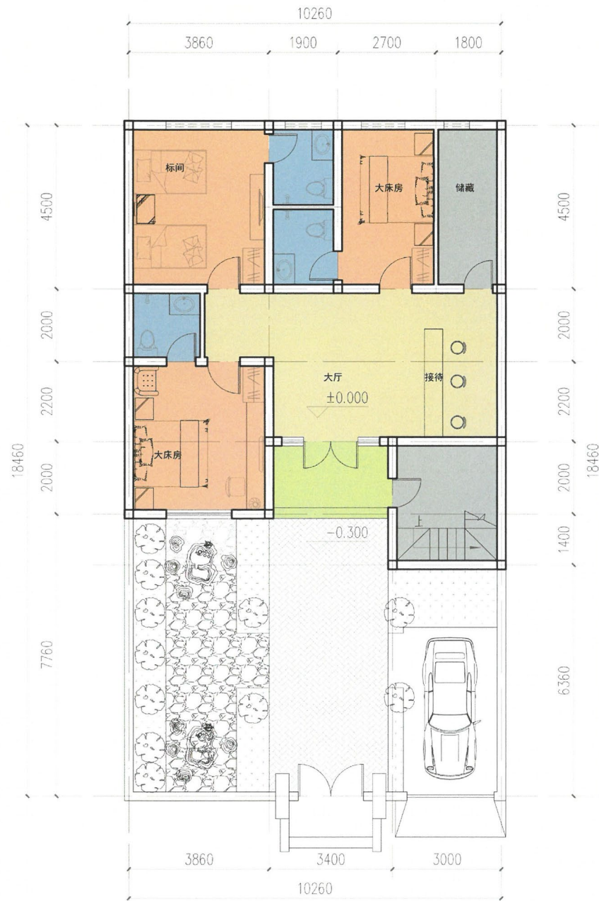
一层平面图
