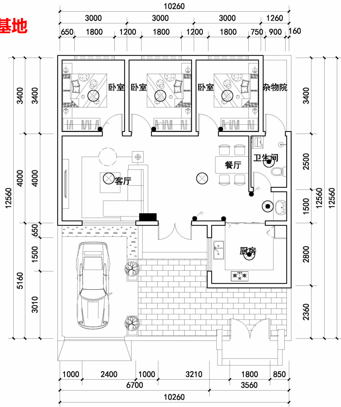
一层照明平面图 1:100
