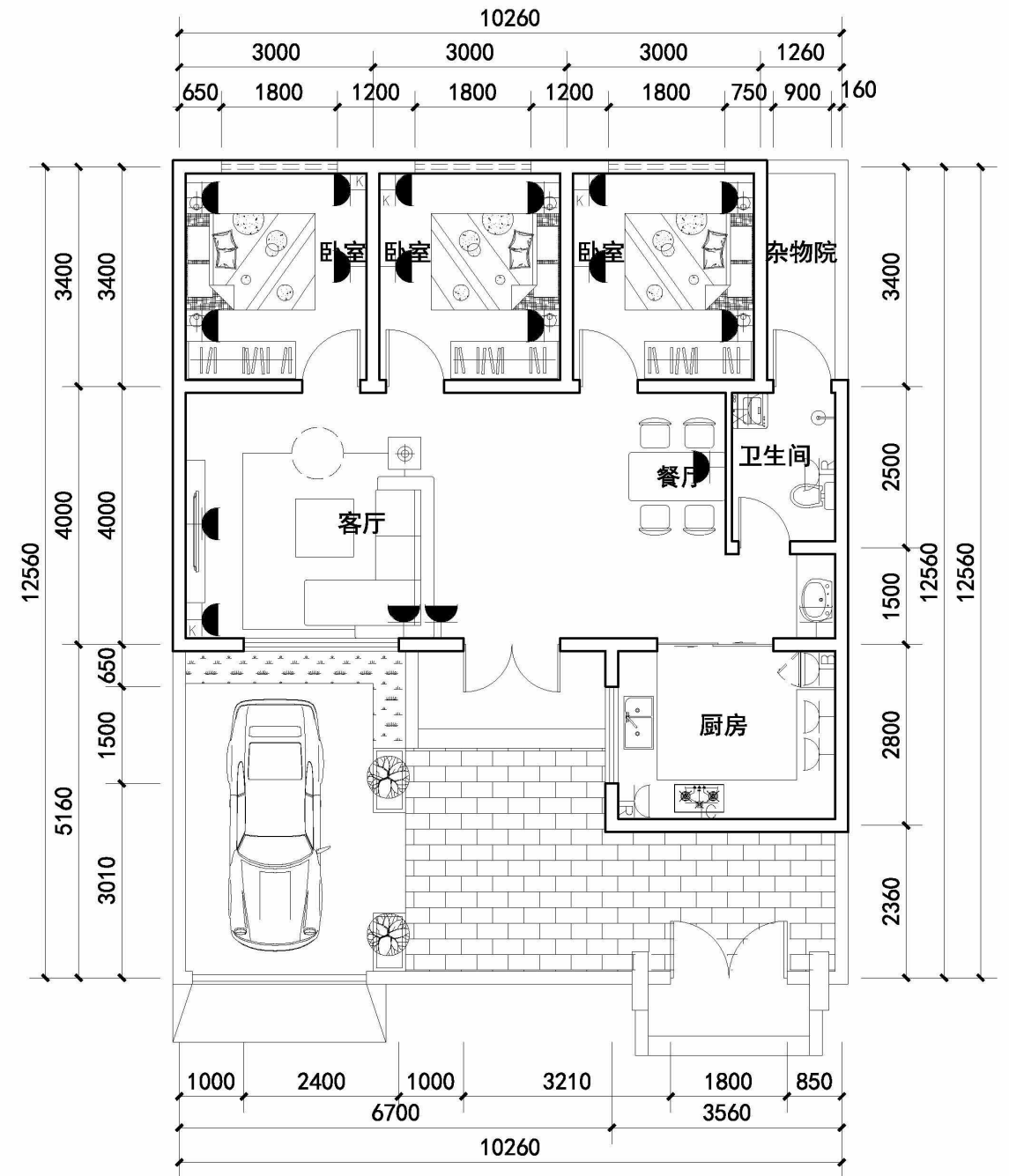
一层插座平面图 1:100
