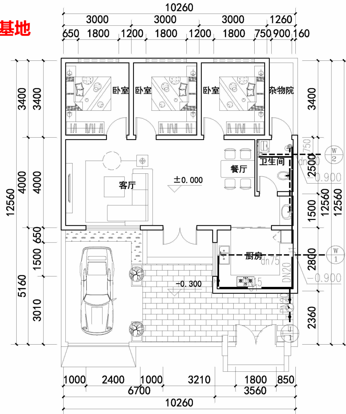
一层平面图 1:100
