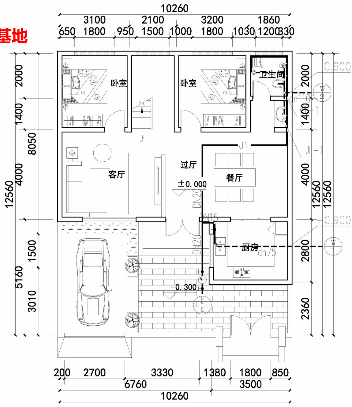
一层平面图 1:100
