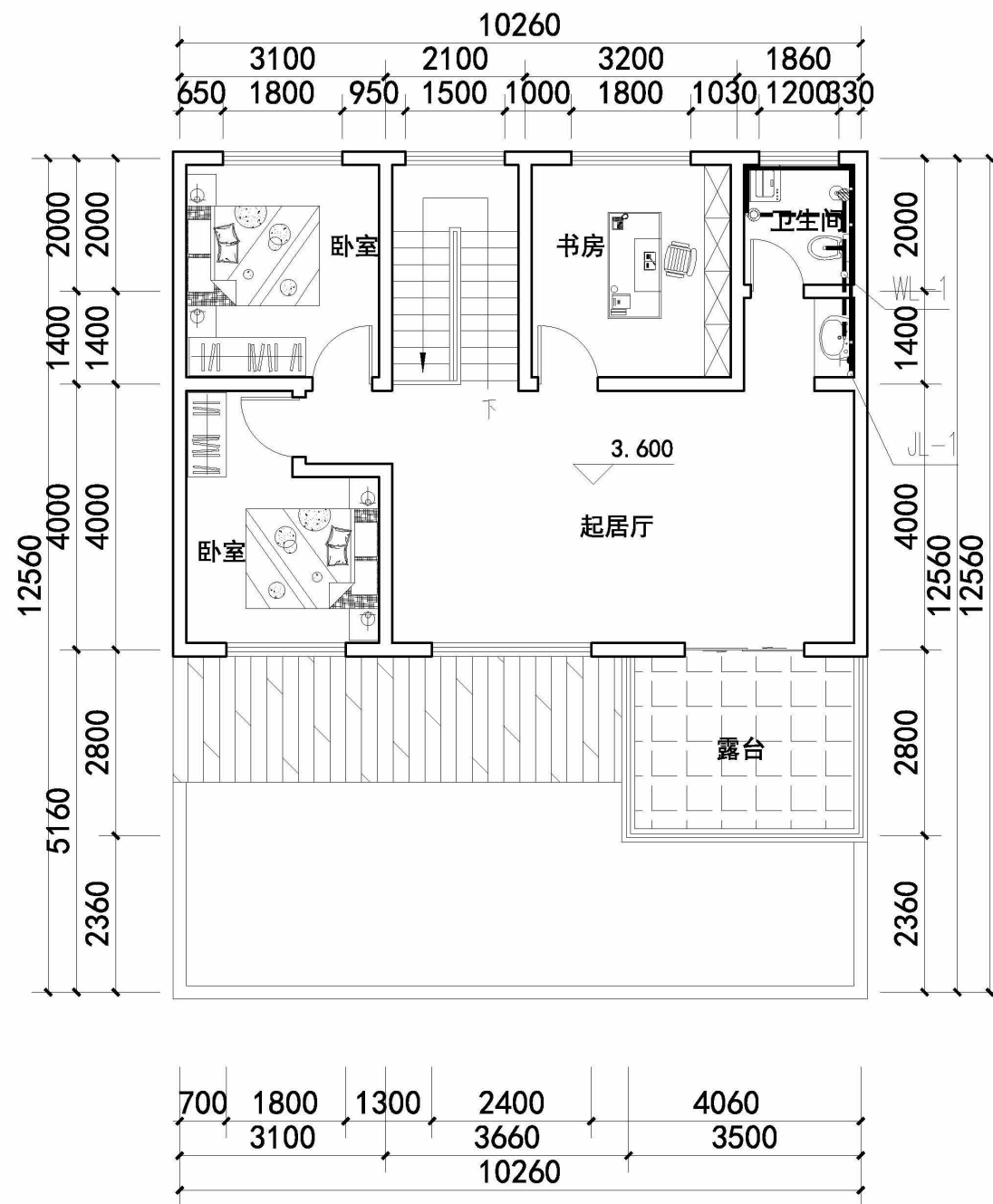
二层平面图 1:100
